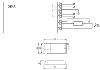
Caractéristiques Philips HID-PV C 50 / I CDM 50/60Hz
