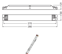
Caractéristiques Osram LED Driver OPTOTRONIC 55/220-240/1A0 CS L G2
